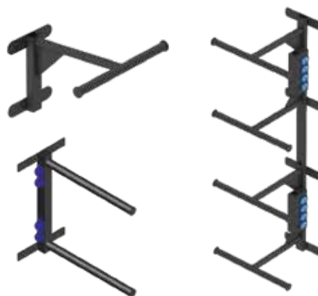
Кронштейны световых прострелов и световых лож
